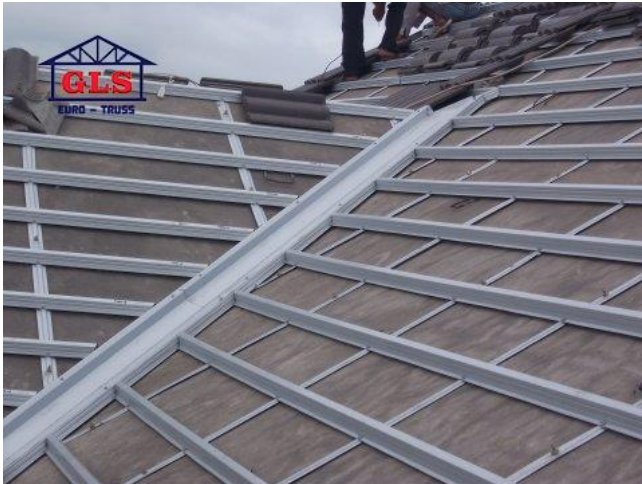
Thép nhẹ Gia Long Steel cho mái bê tông
