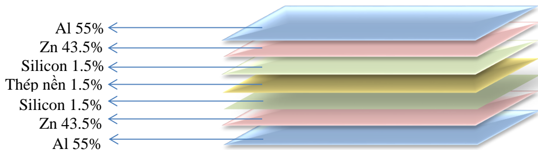
Kết cấu của thép mạ hợp kim nhôm kẽm Euro Truss
